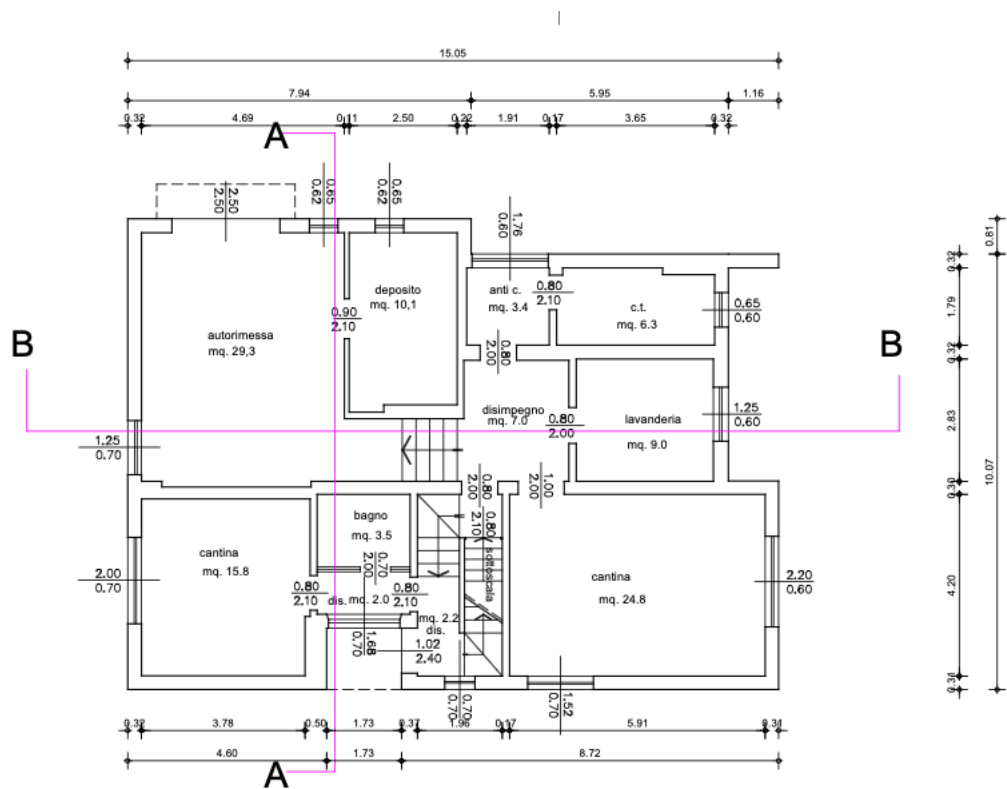
pianta piano seminterrato (terra/interrato)
